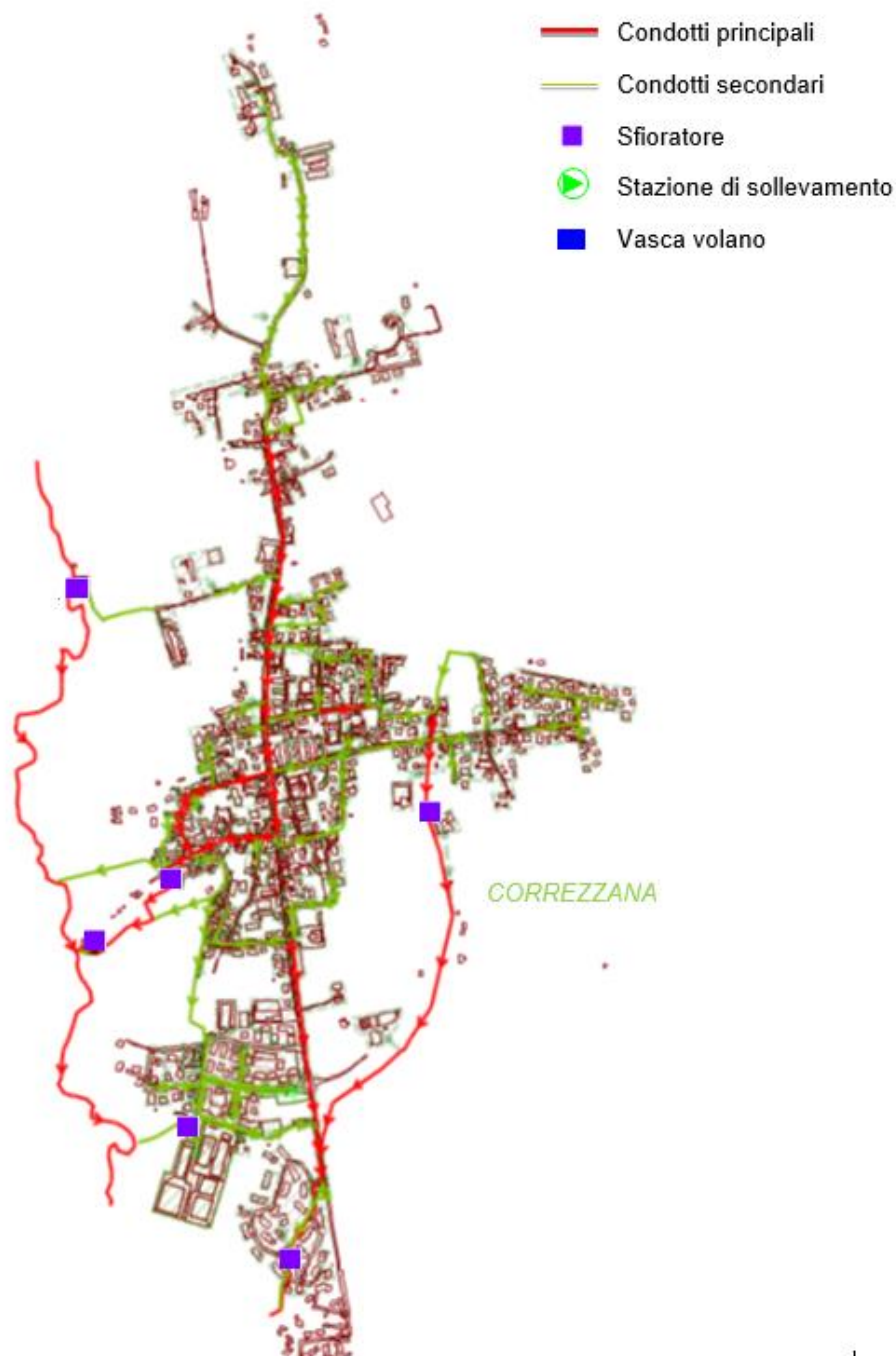
Figura 1: rappresentazione modellistica del sistema di drenaggio integrato
