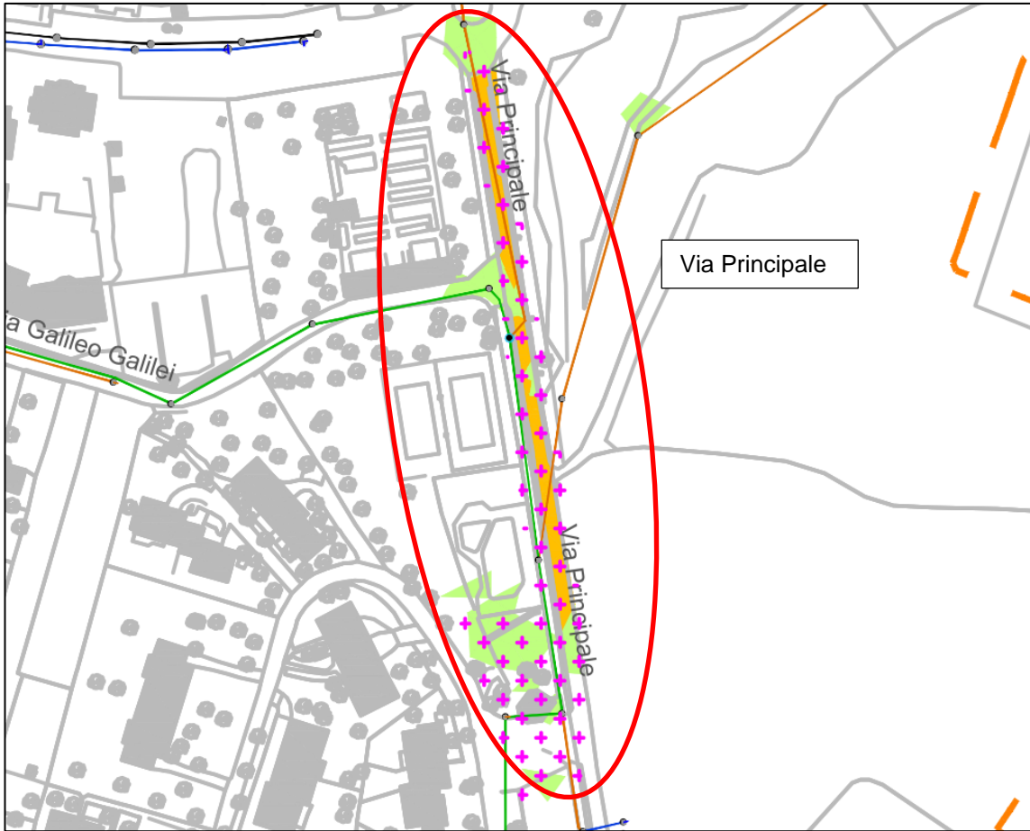
Figura 4: Aree con criticità idraulica dovute alla fognatura e morfologia T50 in Via Principale
